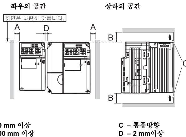
그림 2.3 인버터의 설치공간(열반 : SIDE BY SIDE)
