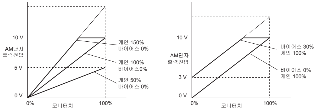
그림 5.29 아날로그 출력의 게인/바이어스 설정
