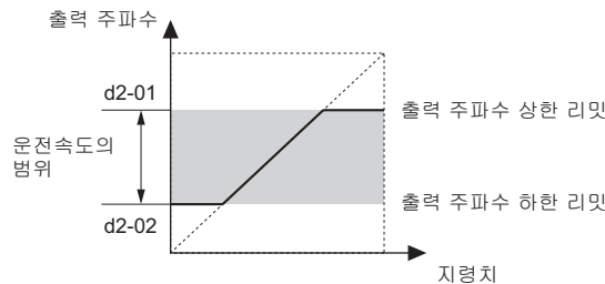
그림 5.8 주파수 지령 상한 · 하한 리미트
