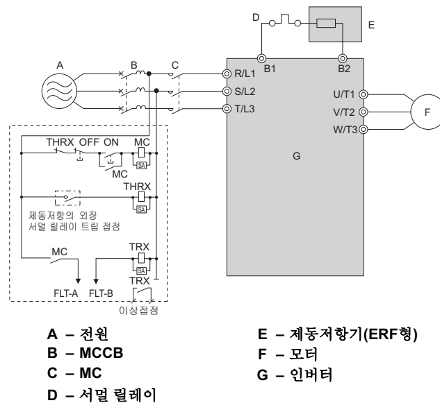
그림 3.21 제동저항기의 접속
