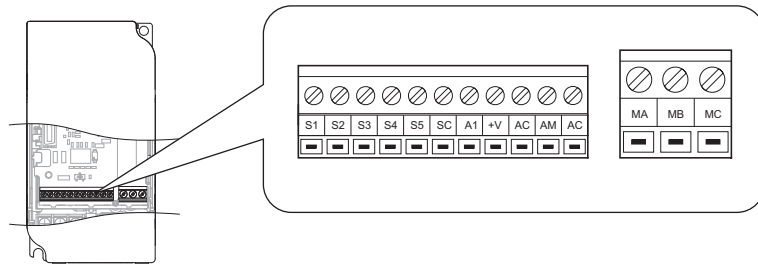
그림 3.11 단자대의 배열
