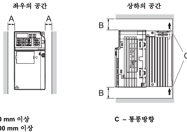
그림 2.2 인버터의 설치공간(단체)
