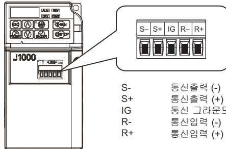
그림 C.2 통신 케이블 접속단자
