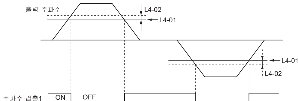
그림 5.20 주파수(FOUT)검출1의 타임차트
