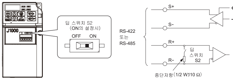
그림 C.5 MEMOBUS통신단자와 DIP스위치S2
