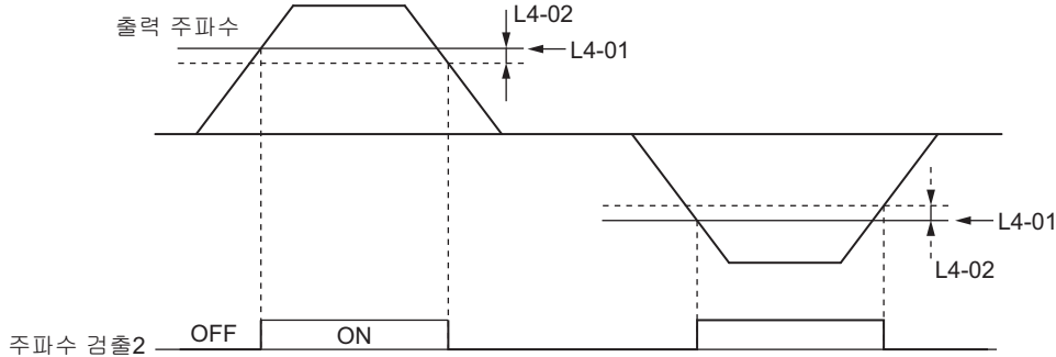
그림 5.21 주파수(FOUT)검출2의 타임차트
