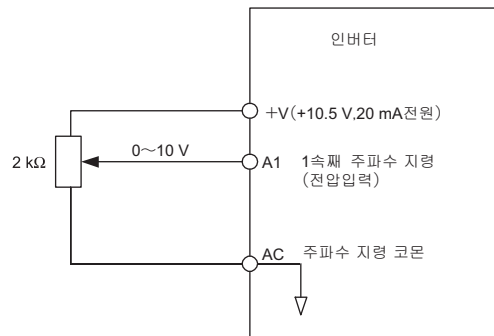
그림 5.1 1속째 주파수 지령의 전압입력
