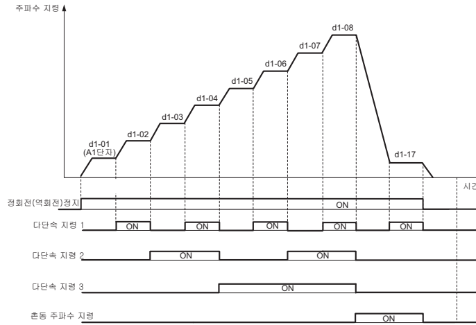
그림 5.7 다단속 지령/촌동 주파수 선택의 타임차트
