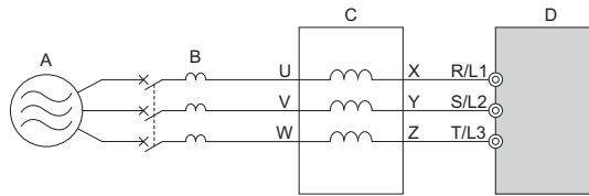
그림 8.4 AC리액터의 접속 예
