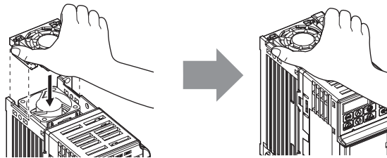
그림 7.4 팬커버의 설치
