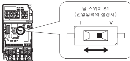
그림 3.20 덤스위치S1
