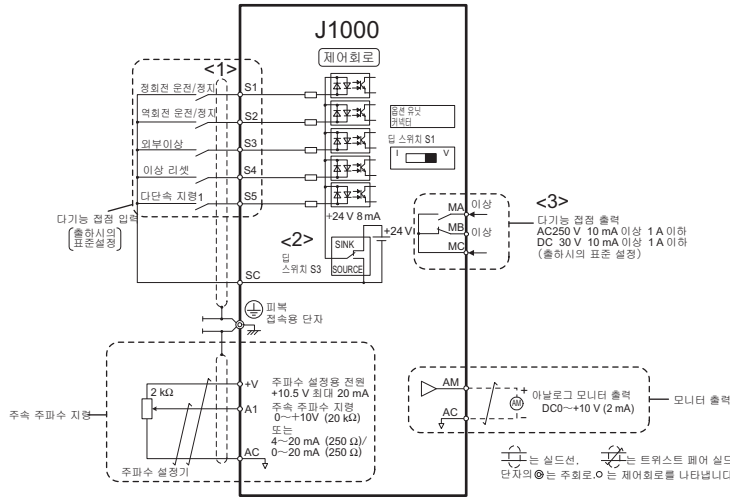
그림 3.10 제어회로 접속도
