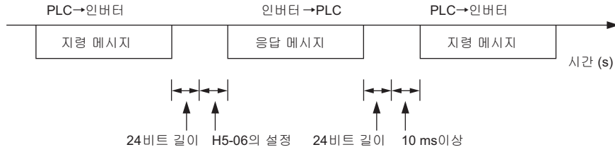
그림 C.6 송신 대기시간
