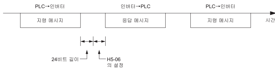
그림 C.8 응답 대기시간
