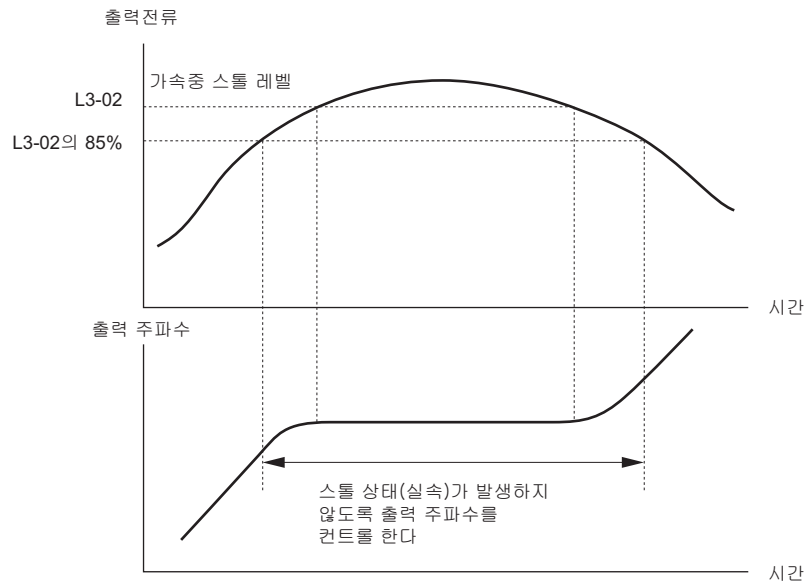
그림 5.32 유도 모터 사용시의 가속중 스톱 방지 기능의 타임차트
