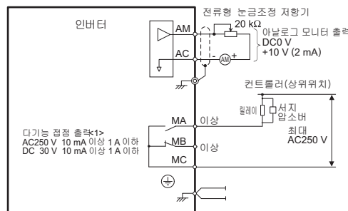
그림 3.19 접점출력
