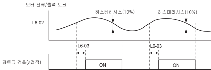
그림 5.36 과토크 검출의 타임 차트
