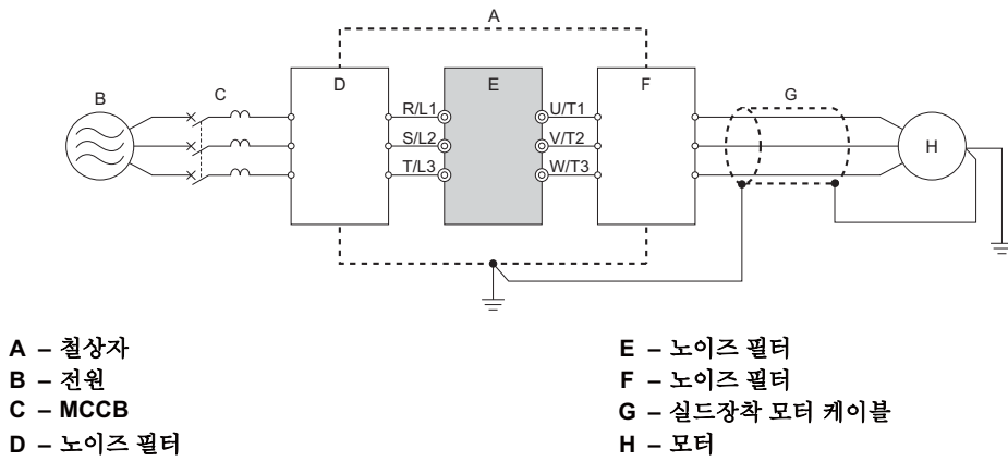
그림 8.10 라디오 노이즈 대책
